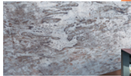
Oberflächenveränderung durch Kondenswasserbildung auf Zinkblech
