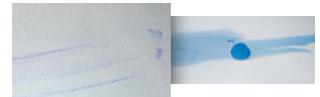
Kein Tintenleck: gute Eloxal-Qualität / Tintenleck: mindere Eloxal-Qualität
