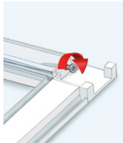
Schraubenfixierung
