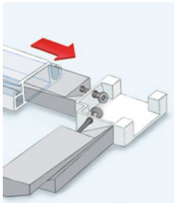
Keile im Eckverbinder sorgen für Halt
