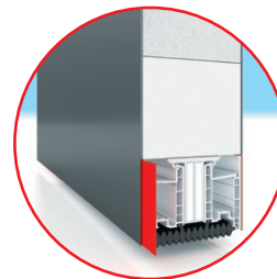
Befestigen von Türpaneelen
